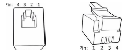
Abbildung 8 Pin – Reihenfolge von RJ 10
