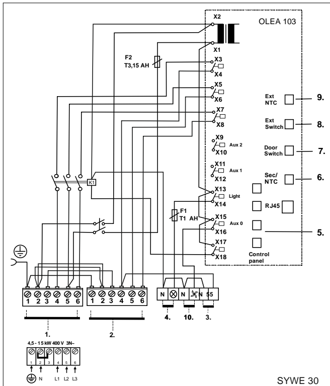
Kuva 10 Kontactori WE 30 ja WE 40 kytkentäkaavat
