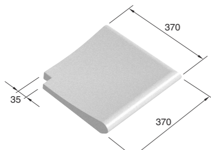
kg 15 Angolo rovescio Inverted angle Angle inversé Randstein rechtwinkliges Außeneckstück
